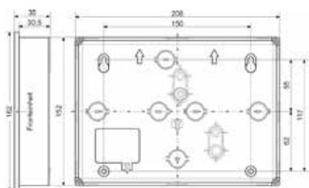
Hluboká zadní stěna
