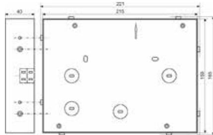
Krabice pro povrchovou montáž
