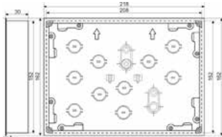
Montážní krabice do duté stěny
